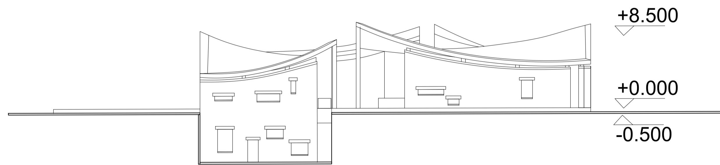
东立面图
