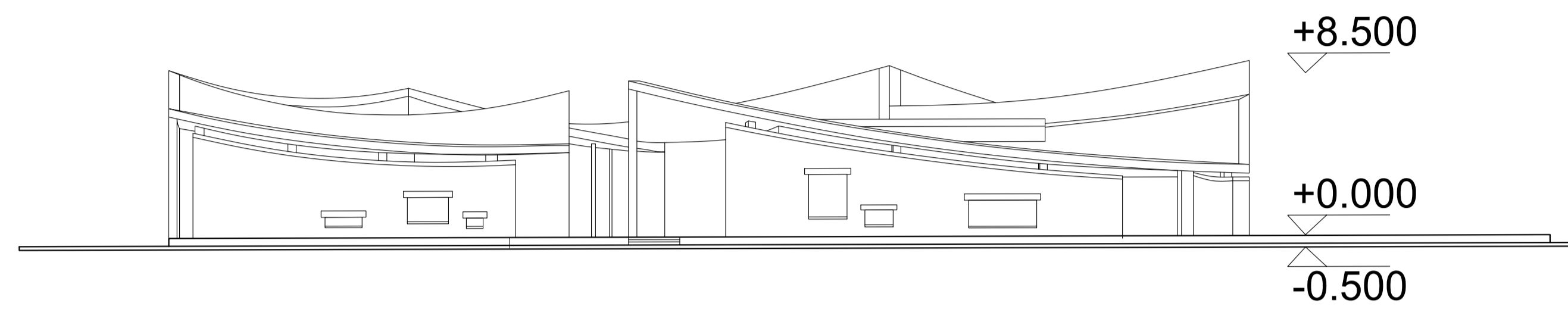
南立面图
