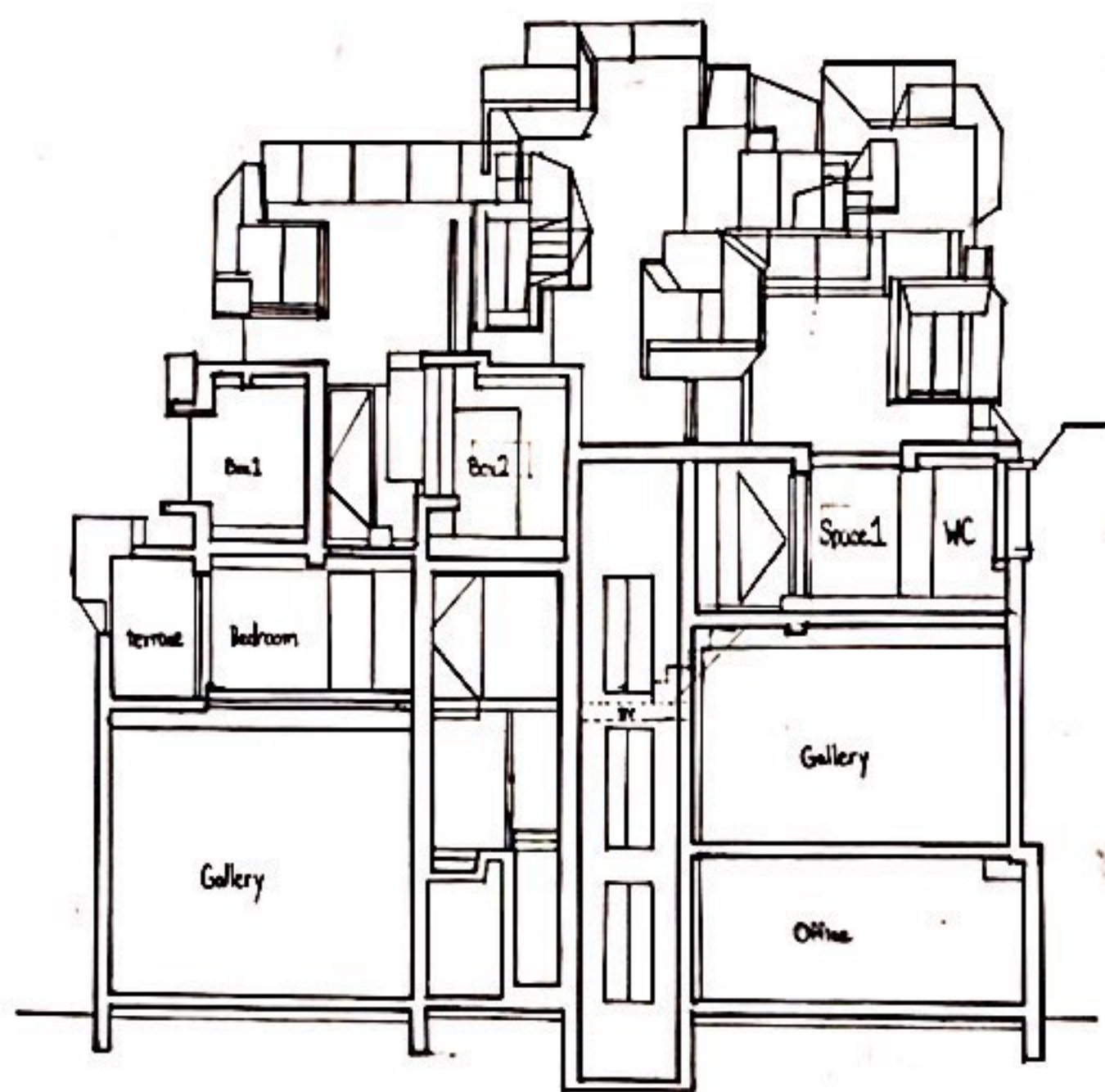
A-A Section
