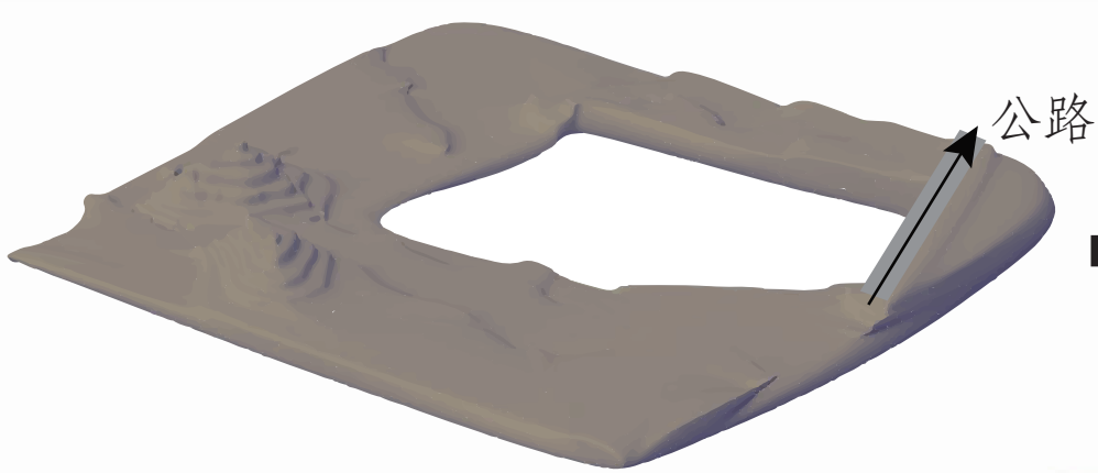
地形模拟
