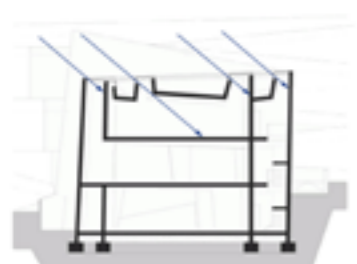
B-B 剖面冬至
