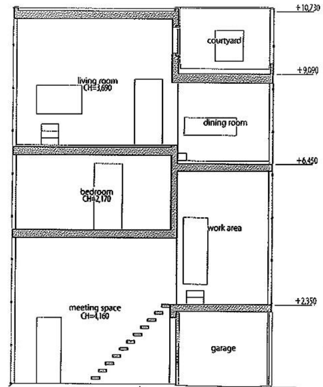
A-A section; scale: 1/150
