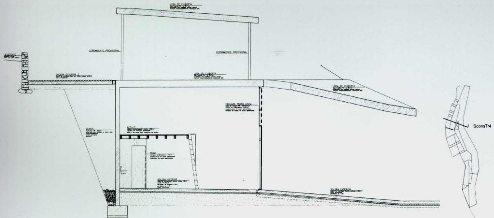
Sección transversal Tr4 / Cross section Tr4
